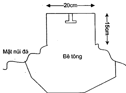
Mốc bê tông gắn trên núi đá
